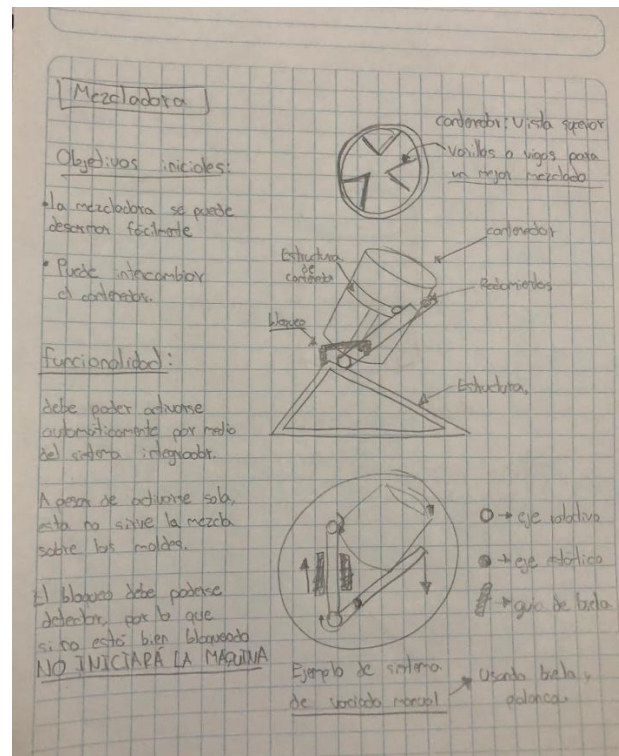
Imagen 1.3 Bosquejo inicial de la mezcladora
