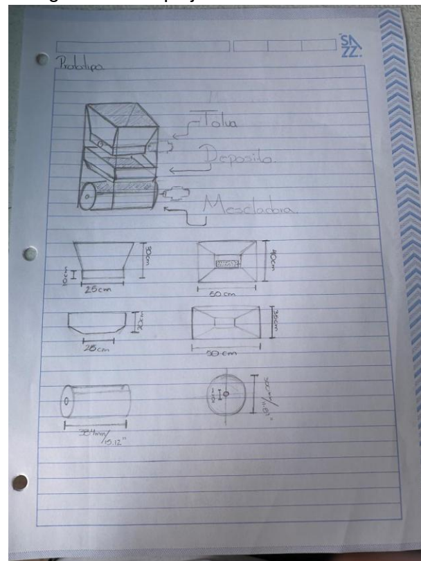
Imagen 1.4 Bosquejo de la mezcladora
